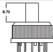
E Extended Actuator
